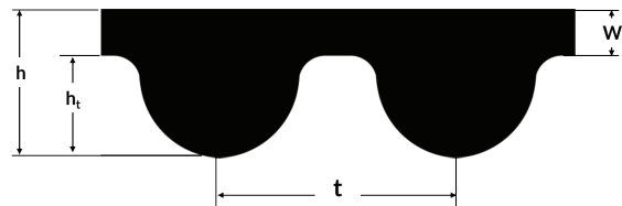
HY-Profil - Zahnform gemäß ISO ISO 13050 [Profile system H]
